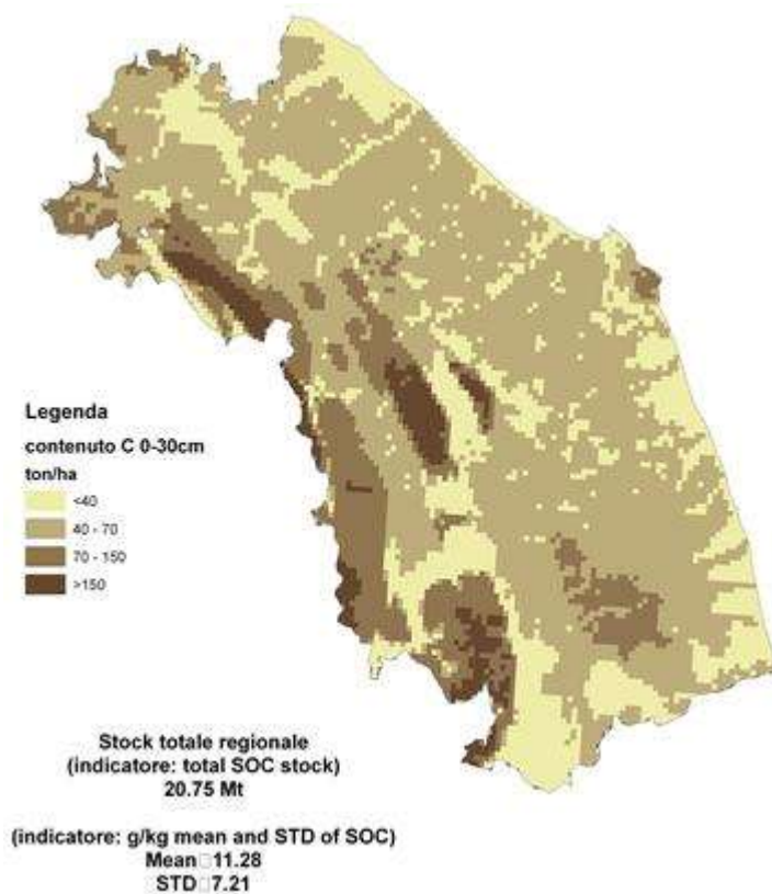
fig.8 - stock di C organico totale regionale
